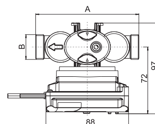
Widok z góry przy montażu przelicznika z boku
