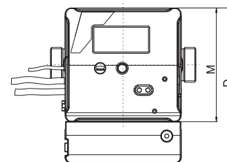
Widok przelicznika zamontowanego na przetworniku
