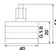
Trójnik DN20 do montażu czujnika temperatury w osłonie
